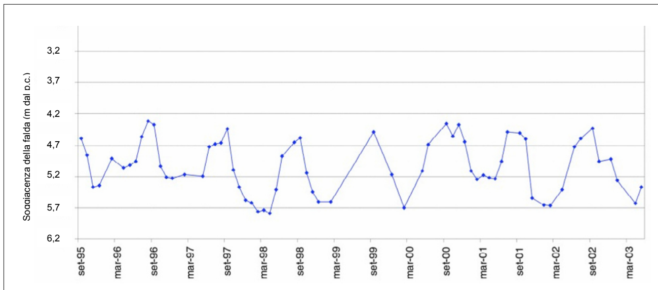
Fig. 8 – Andamento piezometrico nel periodo Settembre 1995 – Marzo 2003 al piezometro T9 installato presso lo stabilimento ex Teksid di Crescentino Rielaborato da: Provincia di Vercelli (2006) – Le acque sotterranee della pianura vercellese
